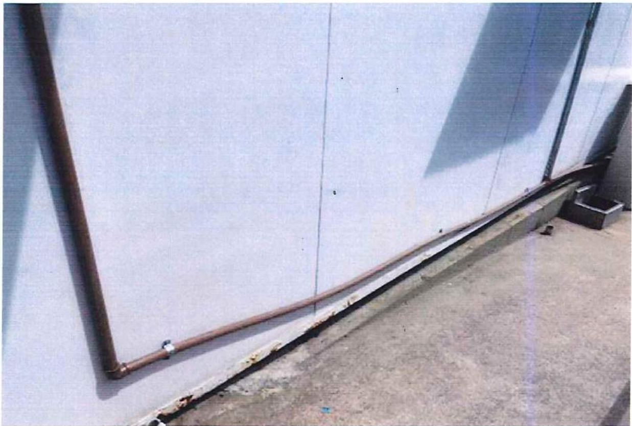
FIGURA 6: Realização de canalização para drenagem e correta destinação de líquido eferente do sistema de refrigeração
